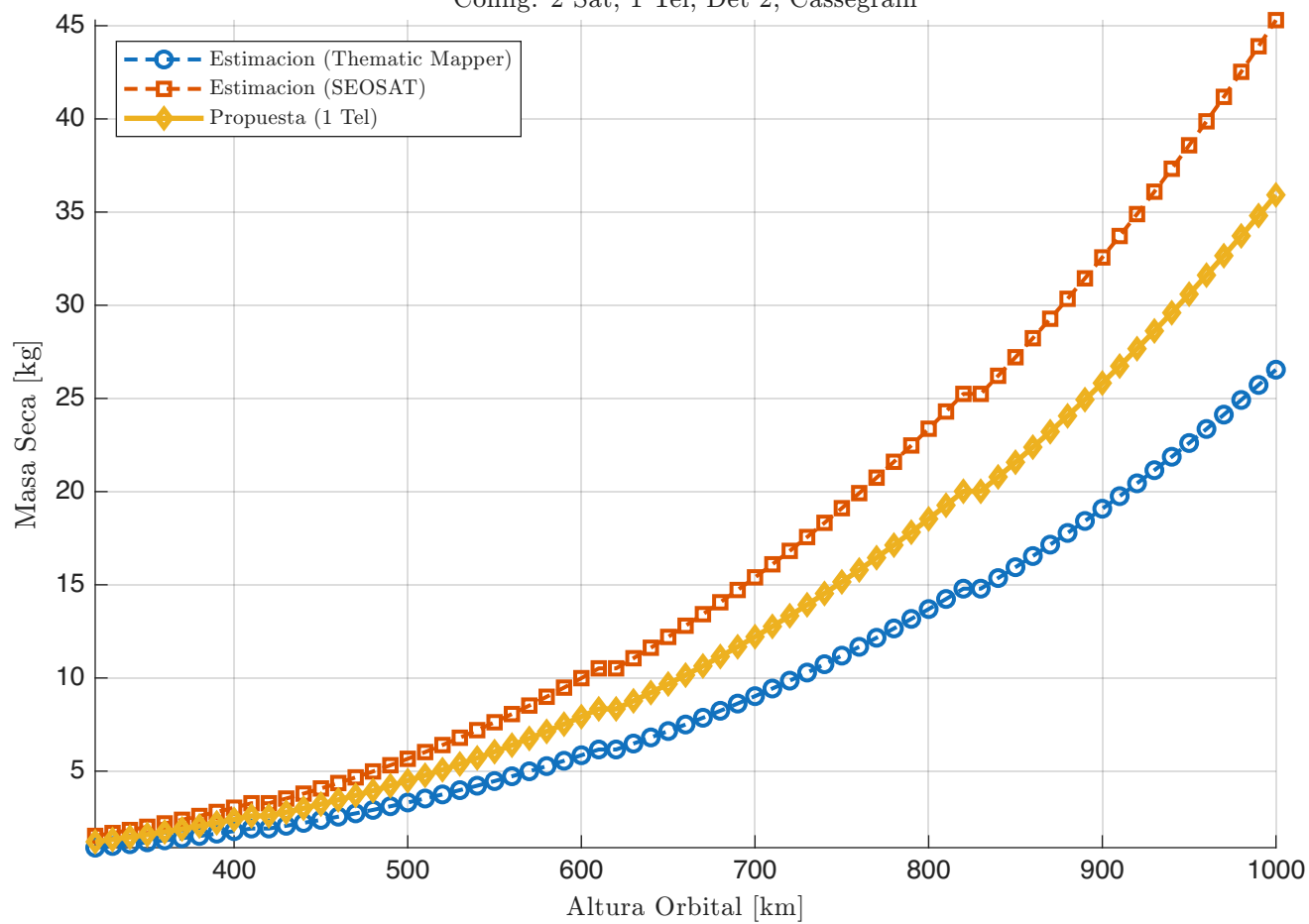
Comparativa de Masa Seca vs. Altura Config: 2 Sat, 1 Tel, Det 2, Cassegrain
